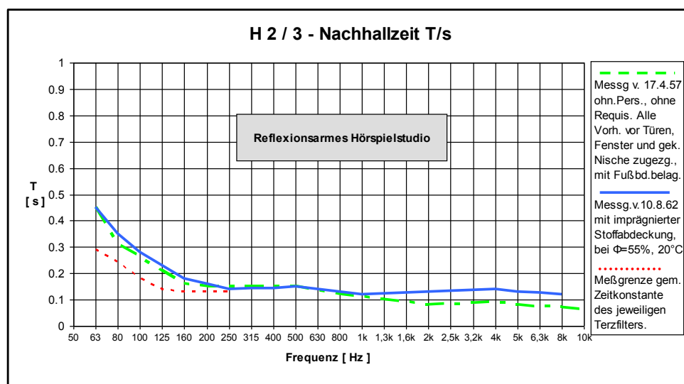
Bild 9.45. Hörspielstudio H 2 / 3. Nachhallzeitverlauf im reflexionsarmen Raum.
