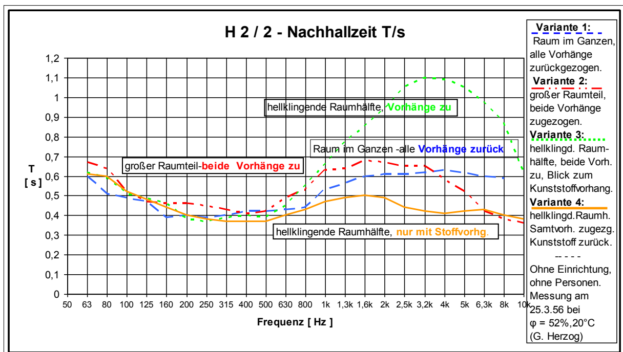
Bild 9.43. Großes Hörspielstudio H 2 / 2: Varianten 1 bis 4 der Nachhallzeitänderungen.
