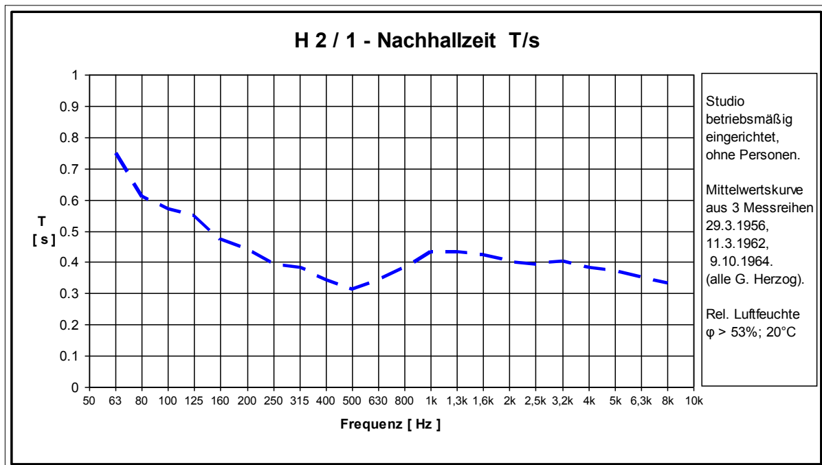
Bild 9.41. Hörspielstudio H2/1 - dunkelklingender Sprecherraum. Nachhallzeitkurve.
